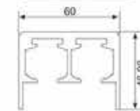
型材截面图
