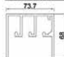
型材截面图
