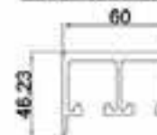
型材截面图
