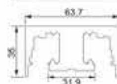
型材截面图
