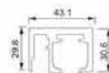
型材截面图
