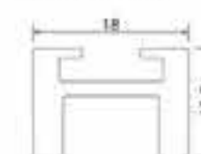
型材截面图
