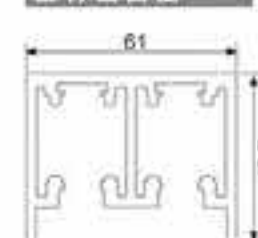
型材截面图
