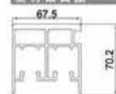
型材截面图
