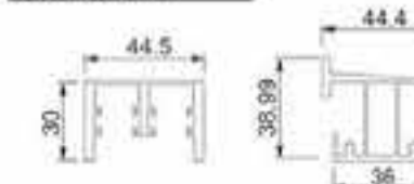
型材截面图
