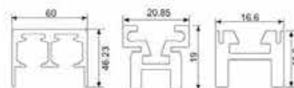
型材截面图
