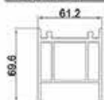
型材截面图
