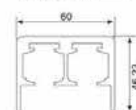
型材截面图
