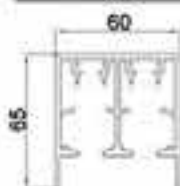
型材截面图
